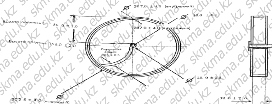
Рисунок 2.9.7-1. Прибор для определения истираемости таблеток Размеры указаны в миллиметрах
